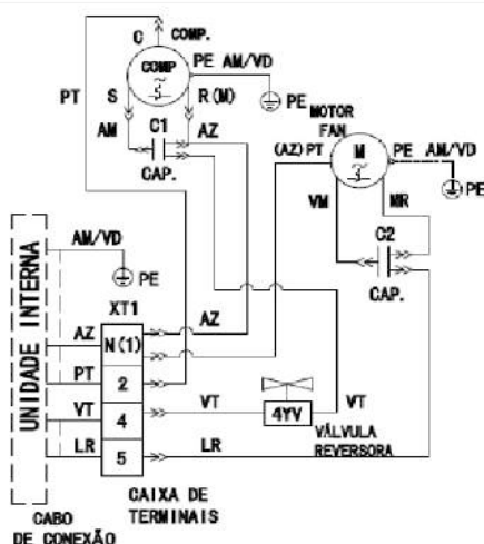
Esquema Elétrico Externo (Quente/Frio): GWH12QC-D3NNB4A (O) GWH18QD-D3NNB4B (O)
