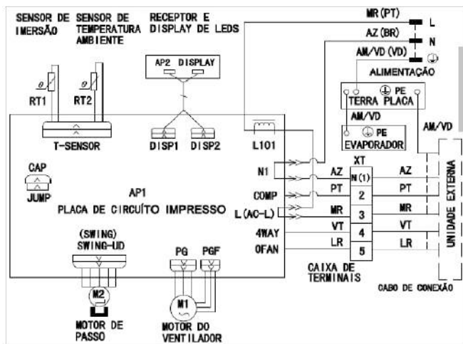
Esquema Elétrico Interno (Quente/Frio): GWH24QE-D3NNB4B (I)
