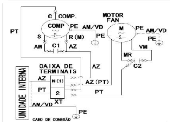
Esquema Elétrico Externo (Frio): GWC09QB-D3NNB4A (O) GWC12QC-D3NNB4A (O)
