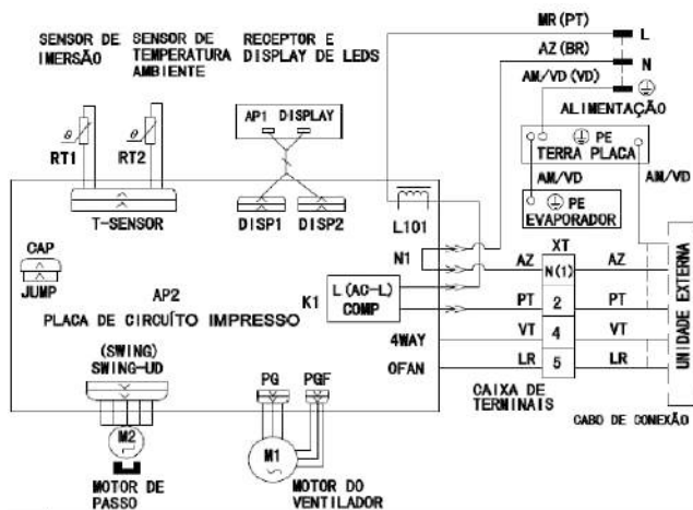
Esquema Elétrico Interno Quente/Frio: GWH18QD-D3NNB4B (I)
