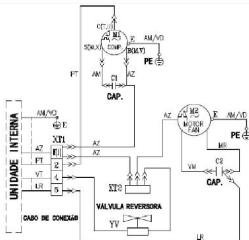
Esquema Elétrico Externo (Quente/Frio): GWH09QB-D3NNB4A (O)
