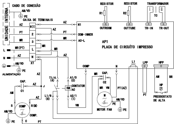
Esquema Elétrico Externo (Frio): GWC24QE-D3NNB4B (O)
