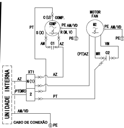
Esquema Elétrico Externo (Frio): GWC18QD-D3NNB4C (O)
