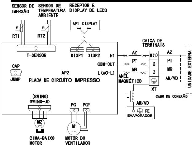
Esquema Elétrico Interno (Frio, Quente/Frio): GWC28QE-D3NNB4B (I) GWH28QE-D3NNB4B (I) GWC30QE-D3NNB4B (I) GWH30QE-D3NNB4B (I)
