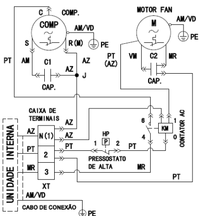
Esquema Elétrico Externo (Frio): GWC24QE-D3NNB4B (O)
