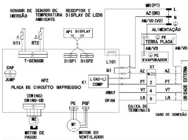
Esquema Elétrico Interno Quente/Frio: GWH18QD-D3NNB4B (I)
